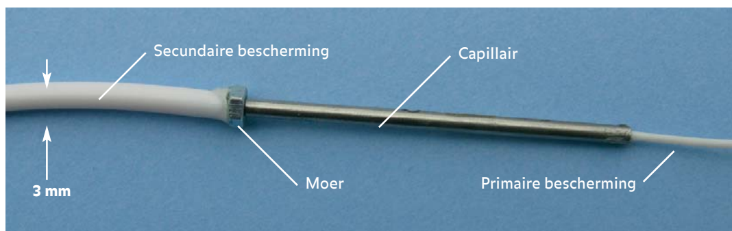
Figuur 7 Foto van een deel van een optische vezel met zicht op de primaire en secundaire bescherming, een capillair en een moerse secundaire bescherming (3 mm).
