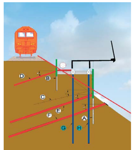
Figuur 2 Detail verstevigings- en funderingsconstructie uitbreidingswerkzaamheden GEN te Ottignies (bron : TUC RAIL n.v.)
