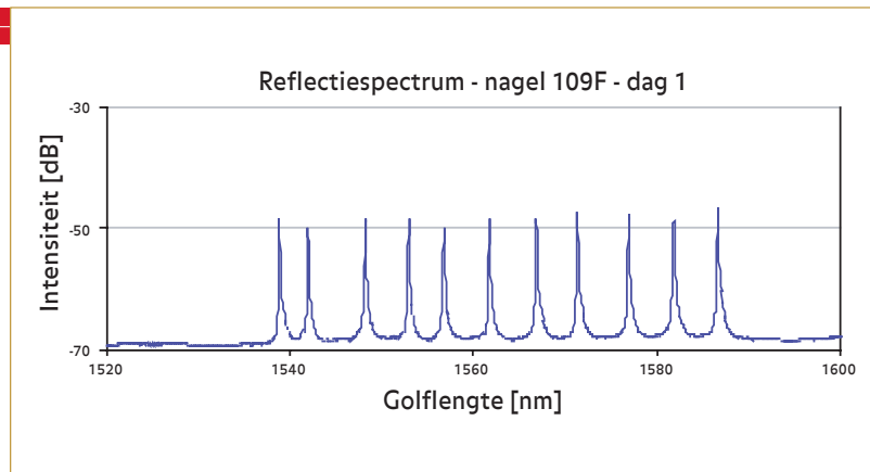
Figuur 5 Het spectrum van het gereflecteerde licht in de optische vezel in nagel 109F op dag 1.
