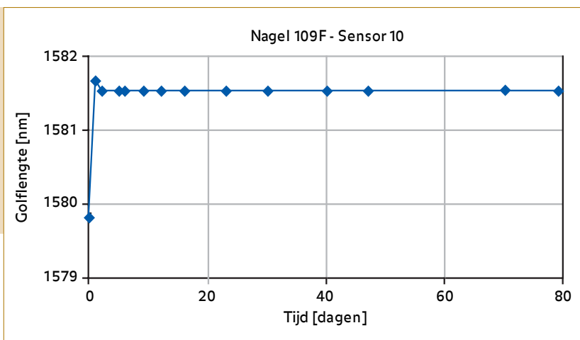
Figuur 12 Evolutie van de metingen van de golflengte [nm] van sensor 10 in nagel 109F in functie van de tijd [dagen] na installatie (installatie = dag 1).
