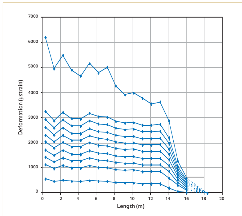
Figuur 8 Belastingsproef (herbelasting t.e.m. stap 9) op holle stang anker te Limelette; vervormingsmetingen met optische vezel met 18 FBG sensoren
