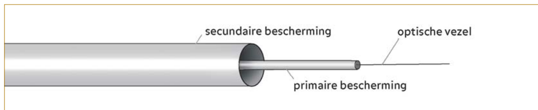
Figuur 6 Schets van de optische vezel (diameter 195 \mu\text{m} ) met een primaire (diameter 900 \mu\text{m} ) en een secundaire bescherming (3 mm).
